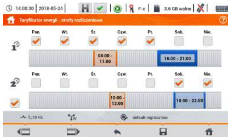
Рис. 6.27 Тарификатор энергии – настройка расчётных зон в зональном тарифе
