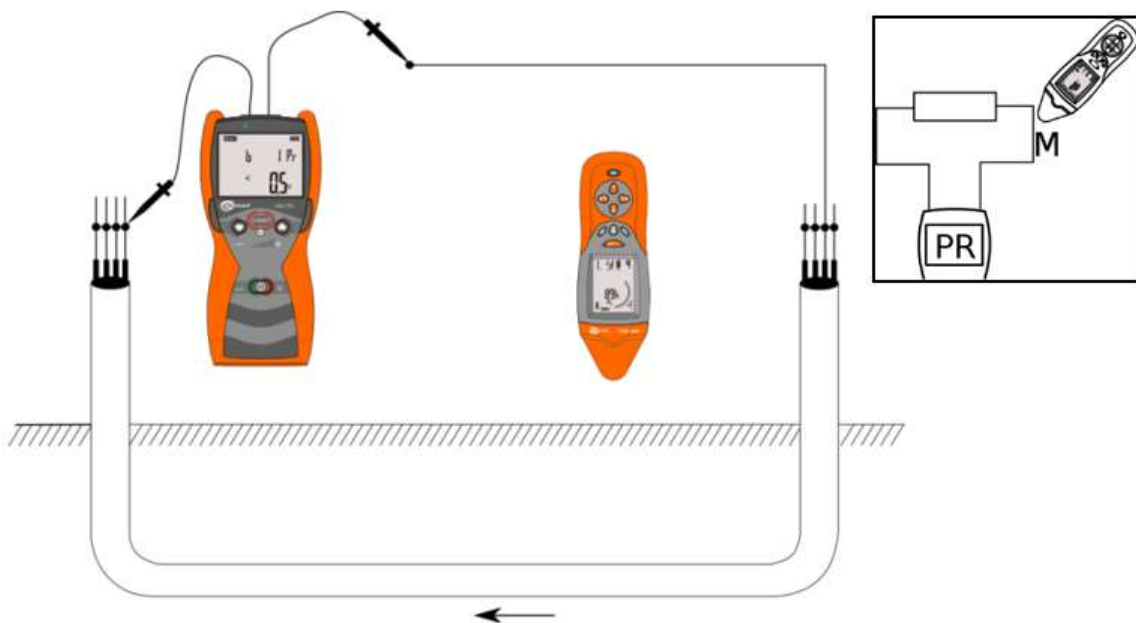
Поиск кабельной линии в режиме « мощность » с помощью внешнего провода
