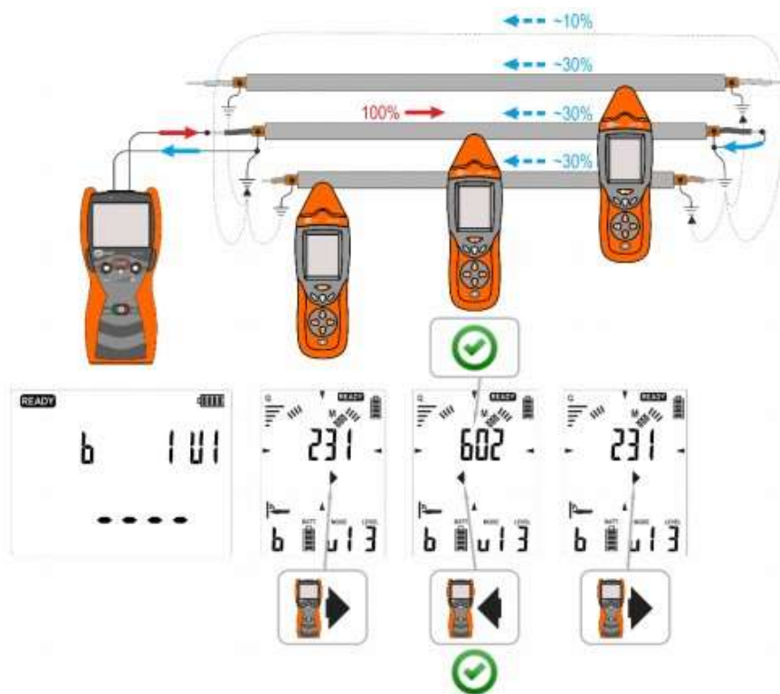
Идентификация кабельной линии с помощью приёмника LKO-720
