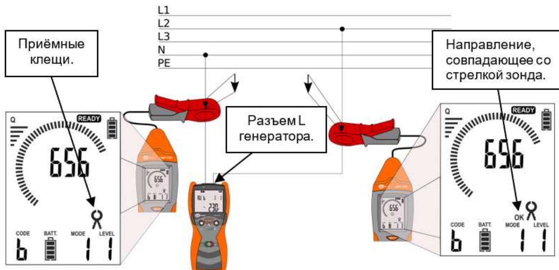
Прохождение токового сигнала в локализованной цепи
